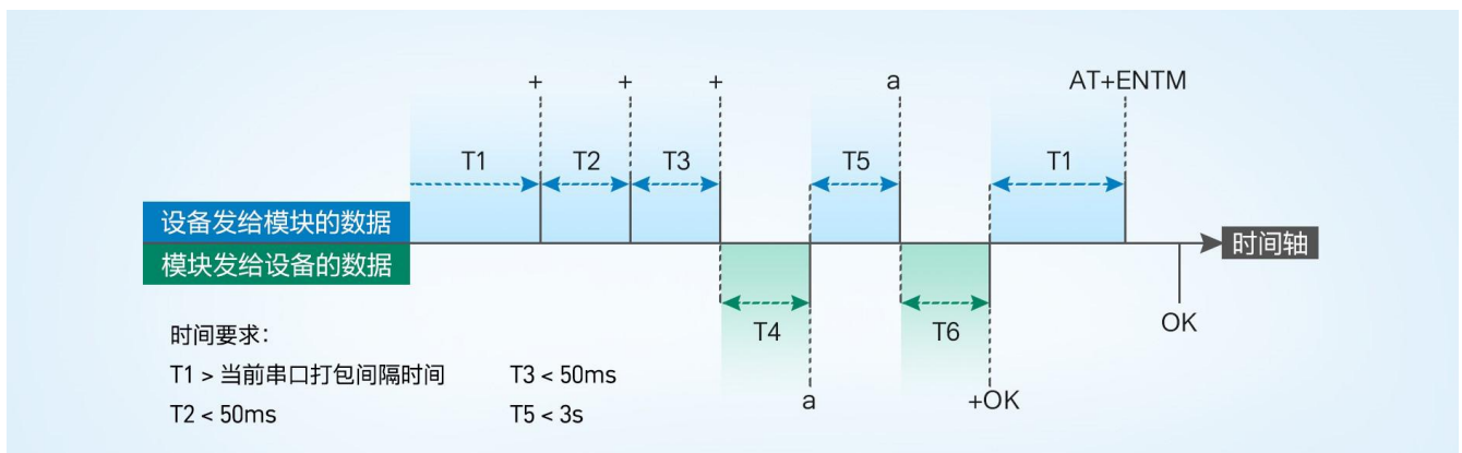
图 28. 切换指令模式时序
