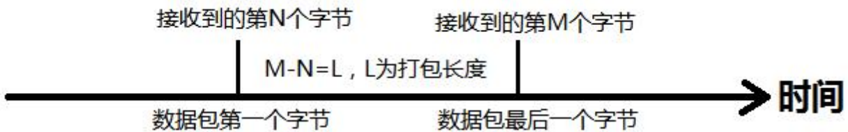
图 27. 长度触发模式
