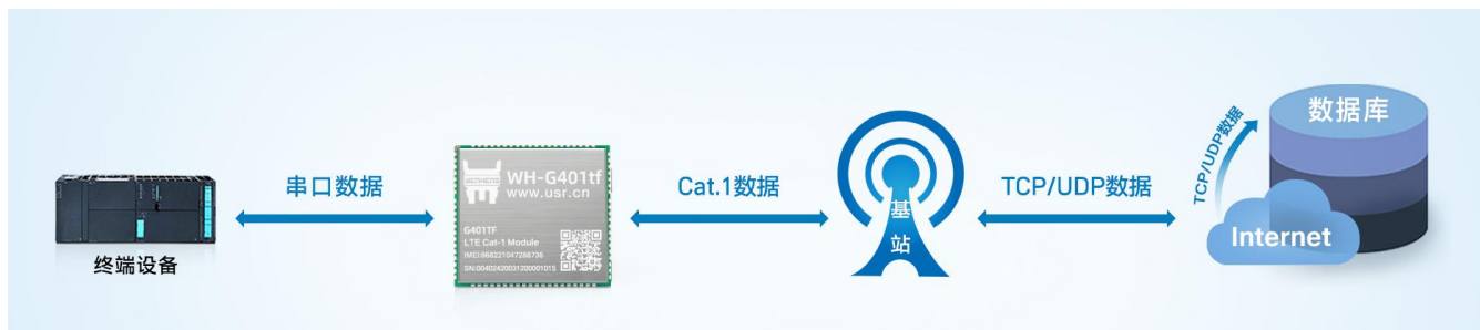
图 1. 测试数据流拓扑图
