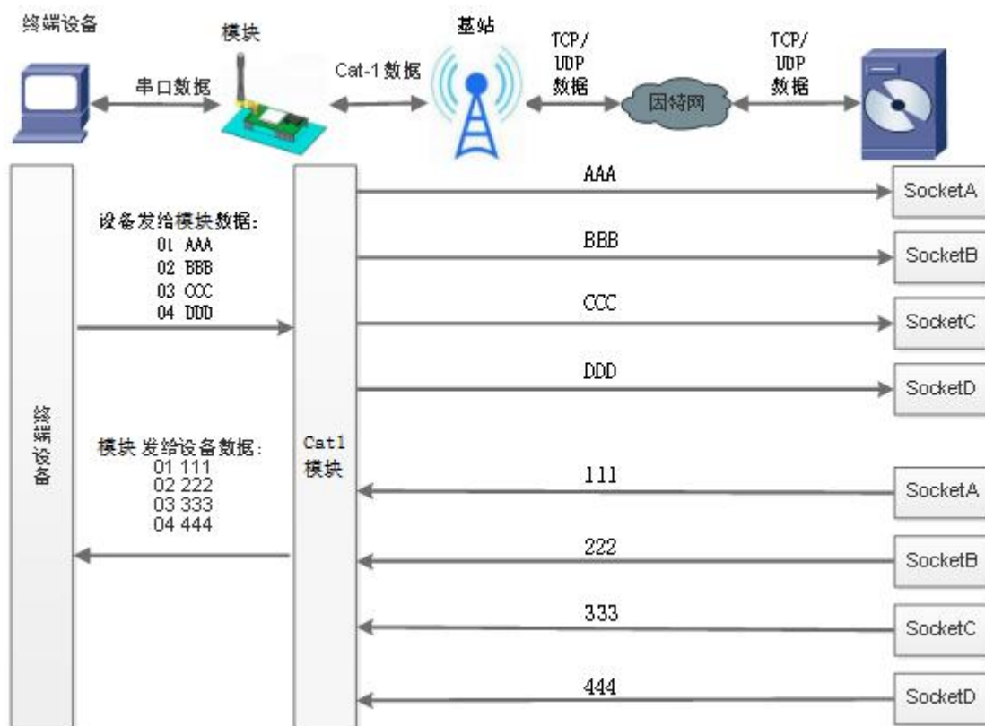
图 14. 套接字分发协议示意图
